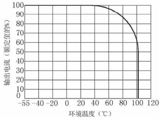
输出电流与环境温度关系曲线
